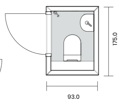
bovenaanzicht toilet 1 e verdieping
